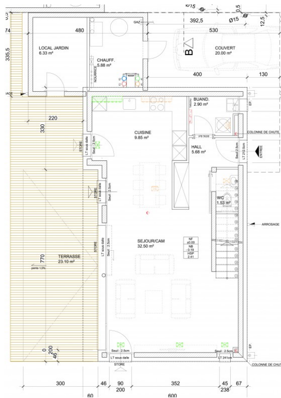
Villa Individuelles "Mnergie" au Bouveret Type B / Rez-de-Chaussée / Ech: 1/50 / RTB Corvaglia Sàrl / 19.06.2015
